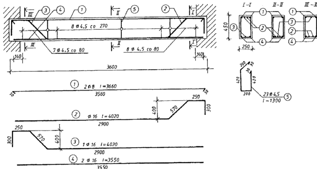
Rys. 48. Wymiarowanie elementów żelbetowych [1, s. 217]
