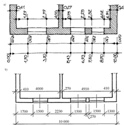
Rys. 60. Rysunek inwentaryacyjny: a) szkic, b) rysunek techniczny fragmentu zinwentaryzowanego pomieszczenia [3, s. 65]
