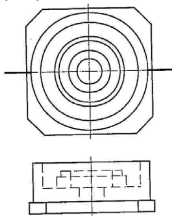
Rys. 49. Rzuty prostokątne przedmiotu o skomplikowanym kształcie [3, s. 44]
