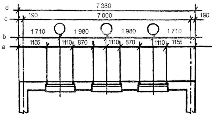
Rys. 46. Przykłady zastosowania ciągów wymiarowych według PN-B-01029:2000
