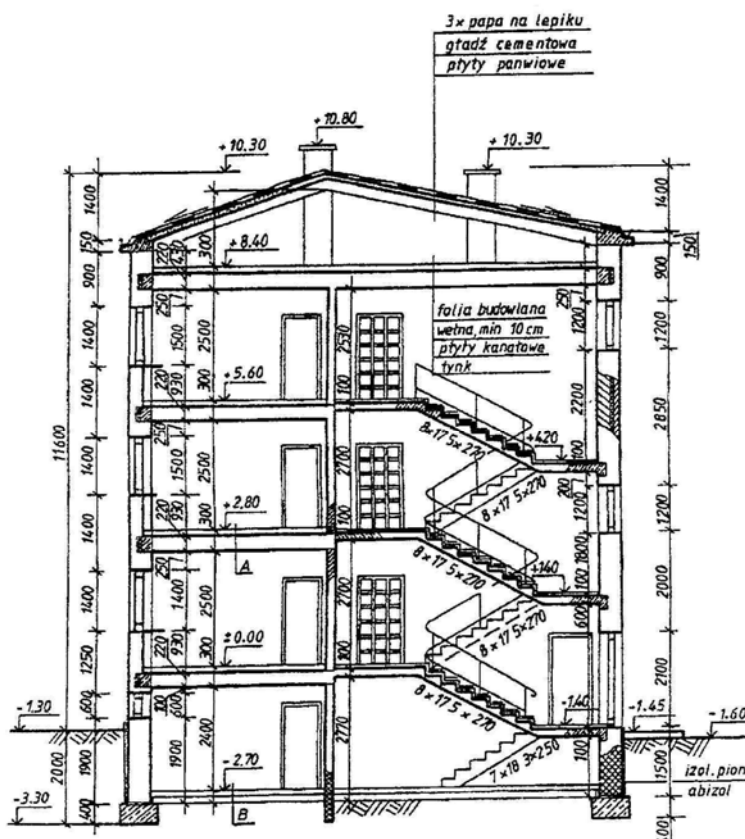
Rys. 55. Przekrój poprzeczny przez budynek według PN-B-01025:2004
