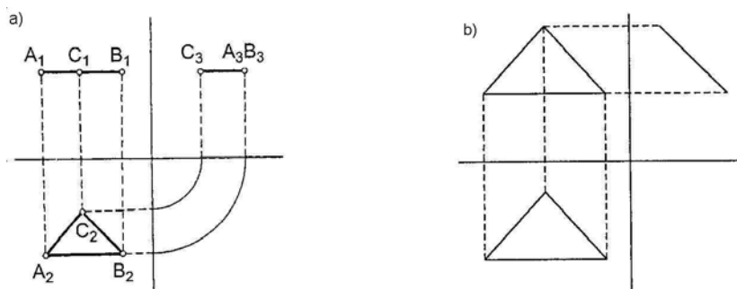
Rys. 12. Rzuty trójkąta: a) równoległego do rzutni poziomej, b) nierównoległego do rzutni [3, s. 23]
