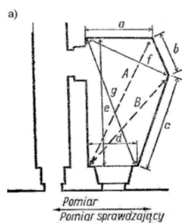
Rys. 61. Pomiar pomieszczenia o rzucie: a) nieregularnym, b) okrągłym [12, s. 111]
