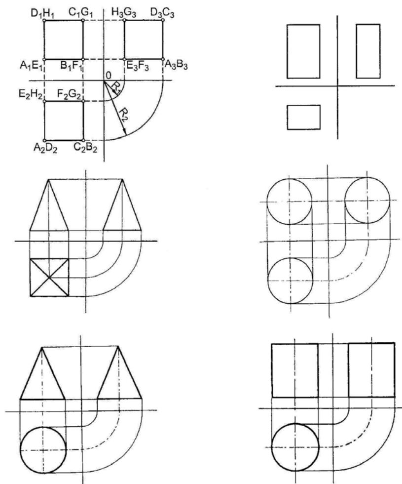
Rys. 17. Rzuty różnych brył na trzy rzutnie [3, s. 24]
