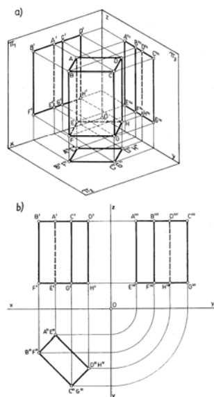
Rys. 16. Rzuty prostopadłościanu, którego ściany boczne nie są ustawione równoległe do rzutni: a) rysunek przestrzenny, b) rysunek rzutowy [17,s. 76]
