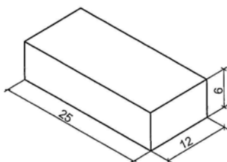
Rys. 44. Pomocnicze linie wymiarowe na rysunku izometrycznym [3, s. 34]
