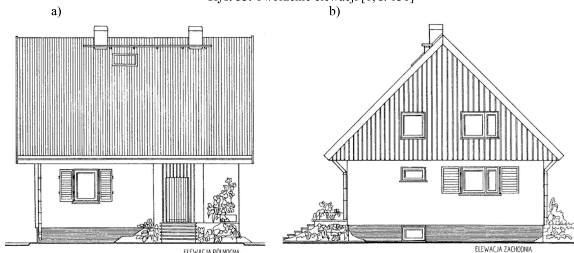
Rys. 54. Elewacje budynku jednorodzinnego: a) północna, b) zachodnia [10, s. 159]
