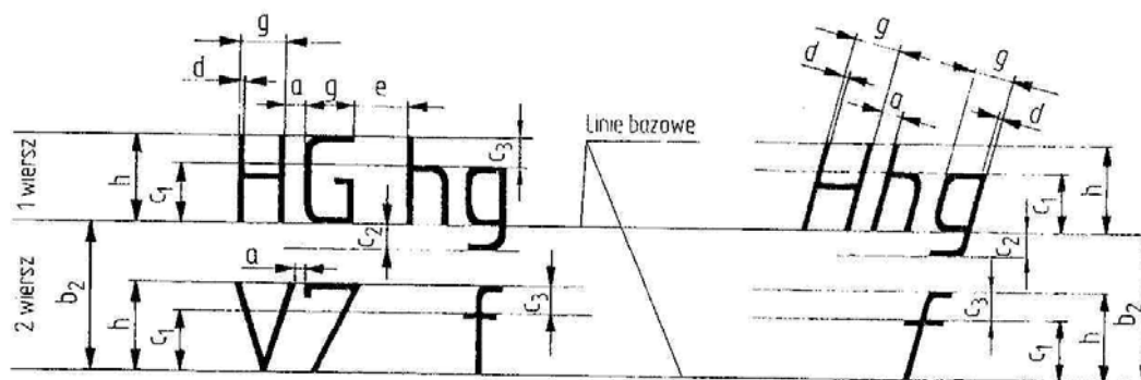
Rys. 42. Elementy prostego i pochyłego odręcznego pisma technicznego [10, s. 22]
