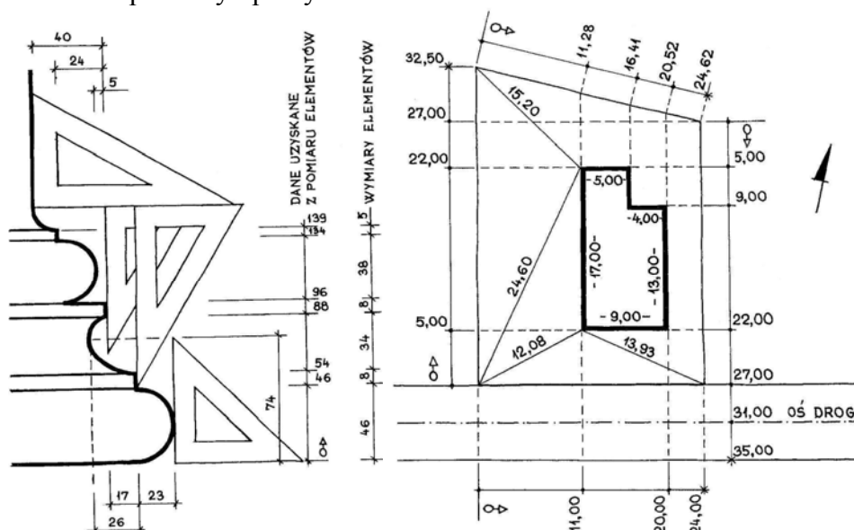
Rys. 63. Inwentaryzacja detalu architektonicznego i działki budowlanej [2, s. 145]
