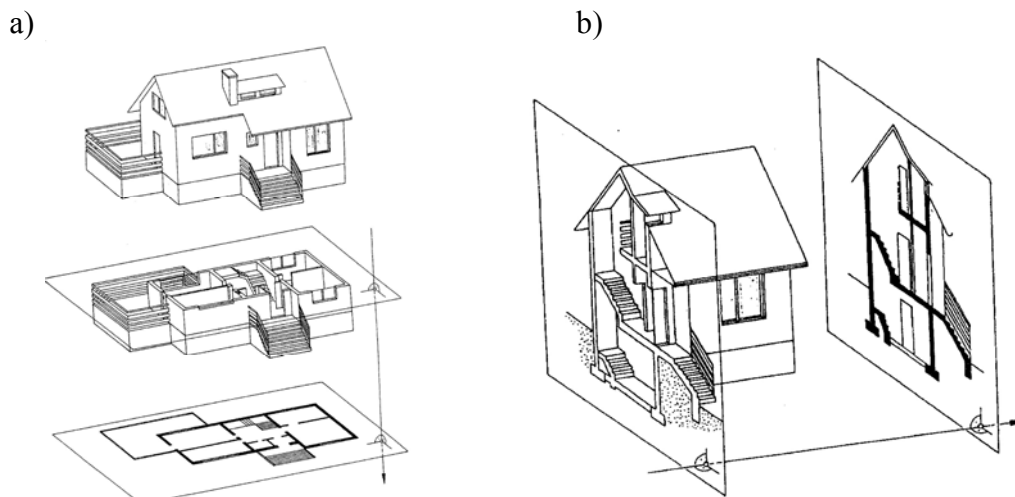
Rys. 50. Tworzenie przekrojów budynku: a) poziomego, b) pionowego [1, s. 135]
