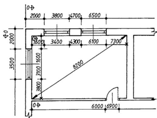
Rys. 59. Szkic inwentaryacyjny pomieszczenia [1, s. 170]
