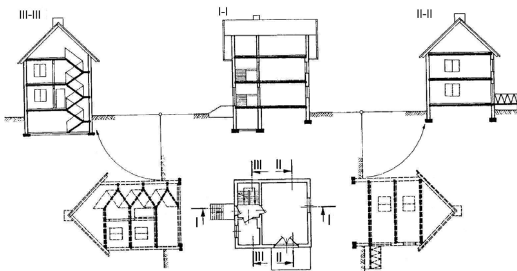
Rys. 51. Zasada oznaczania przekrojów budynku [17, s. 86]
