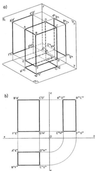
Rys. 15. Rzuty prostopadłościanu, którego ściany są ustawione równoległe do rzutni: a) rysunek przestrzenny, b) rysunek rzutowy [17,s. 76]
