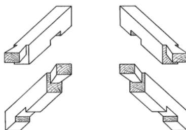
Rys. 7. Rysunek elementów budowlanych w aksonometrii ukośnej kawalerskiej o współczynniku deformacji liniowej [17, s. 53]
