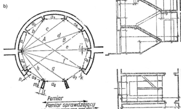
Rys. 61. Pomiar pomieszczenia o rzucie: a) nieregularnym, b) okrągłym [12, s. 111]
