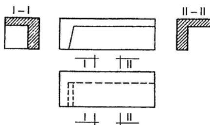
Rys. 29. Przykład rysowania przekrojów ze wskazaniem kierunku patrzenia [3, s. 47]
