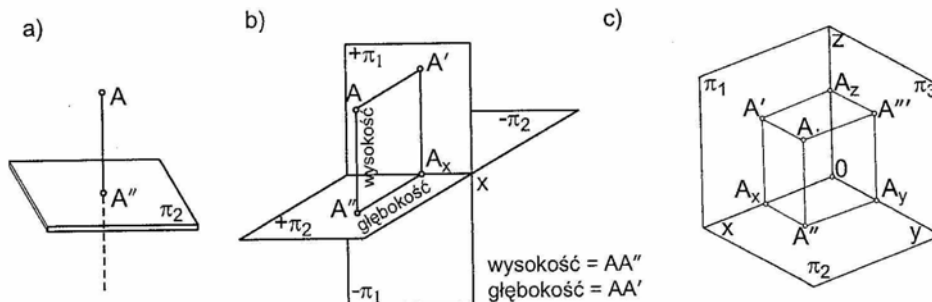
Rys. 9. Rzutowanie punktu A na jedną (a), dwie (b) i trzy płaszczyzny [3, s. 22]
