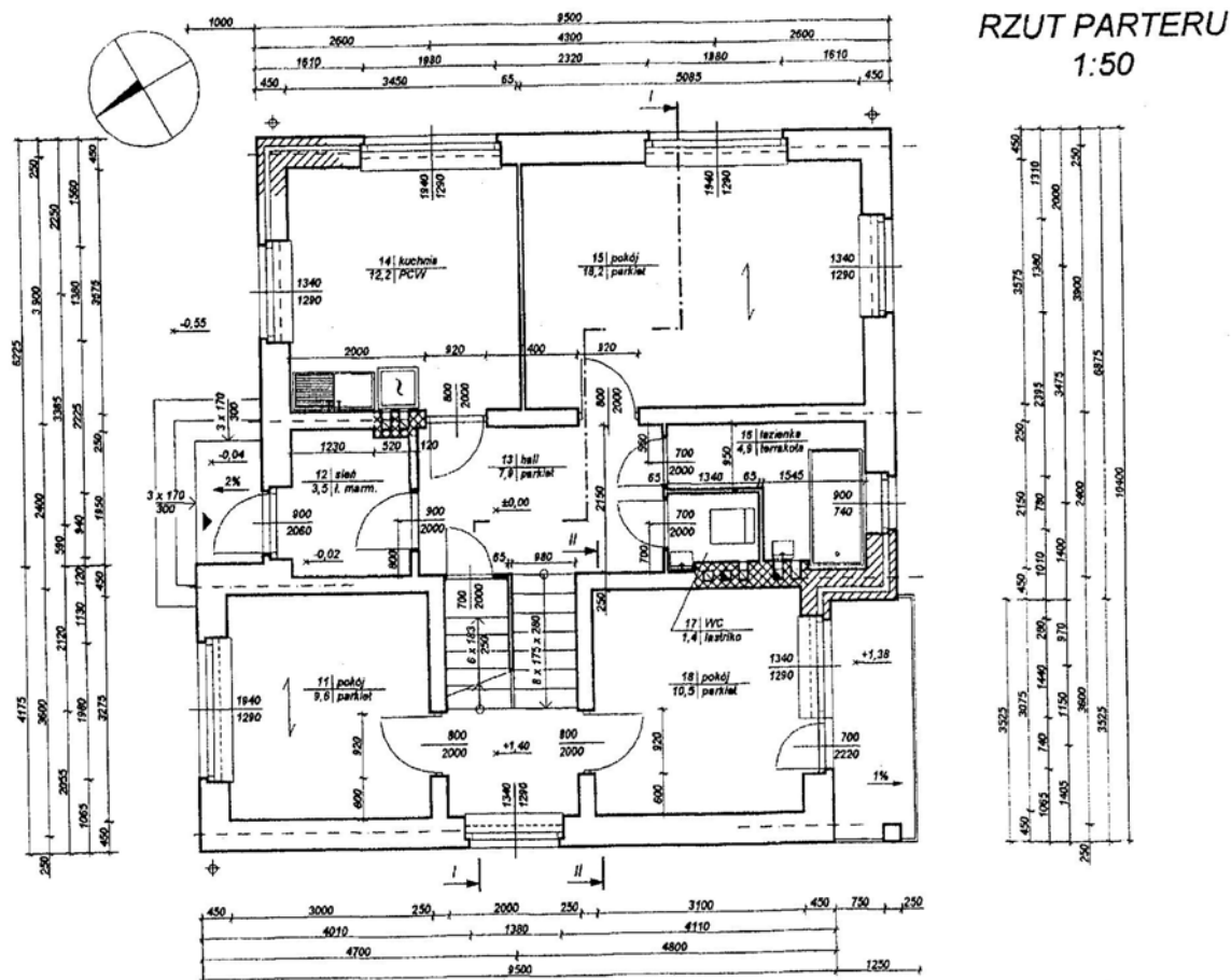
Rys. 52. Rzut parteru budynku jednorodzinnego [1, s. 188]
