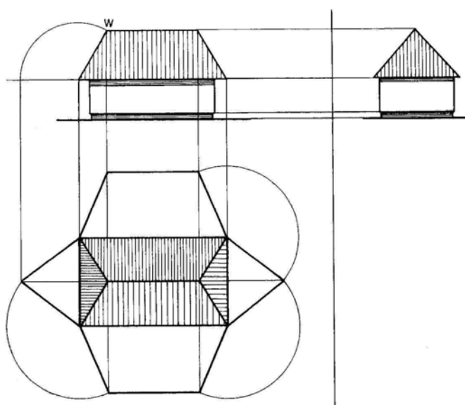
Rys. 34. Rozwinięcie połaci dachu [17, s. 94]
