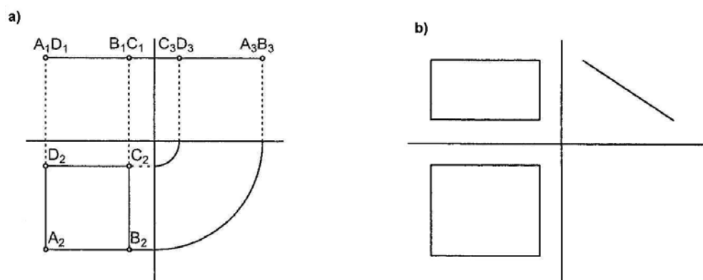
Rys. 13. Rzuty kwadratu: a) równoległego do rzutni poziomej, b) nierównoległego do rzutni [3, s. 23]
